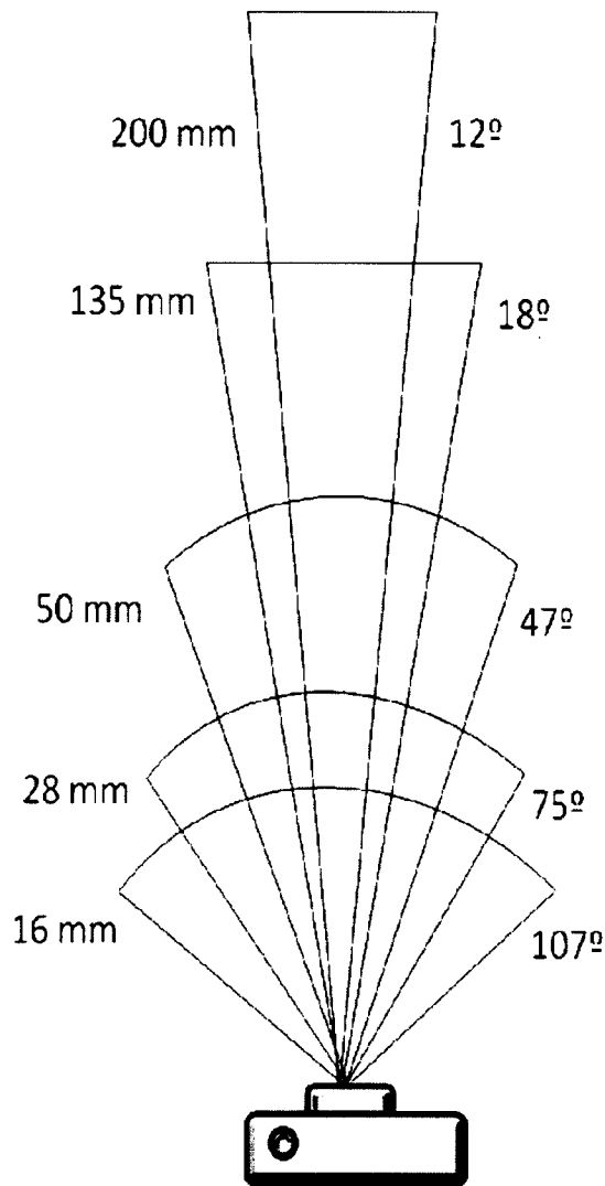
圖 17 攝影鏡頭規格與功率
