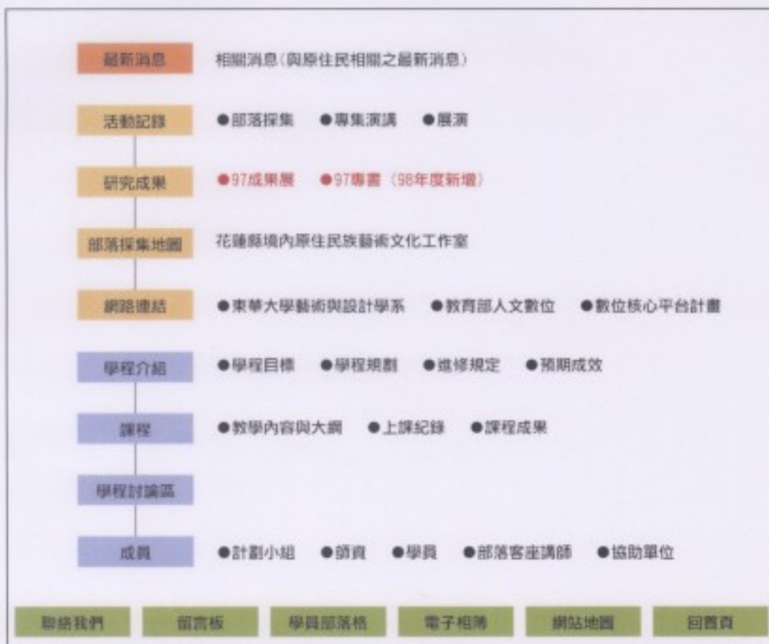
圖 1 網頁架構圖
