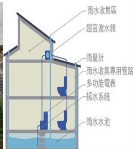
(c)大樓雨水回收系統圖
