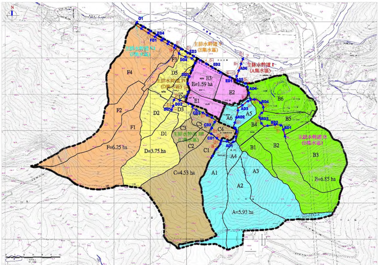
圖5 雙溪校區主要排水幹道分布圖
