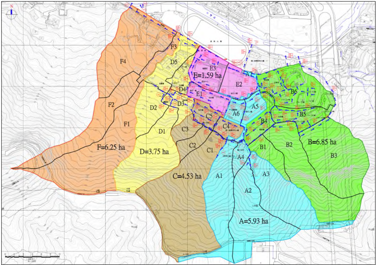
圖4 雙溪校區現況排水調查結果圖
