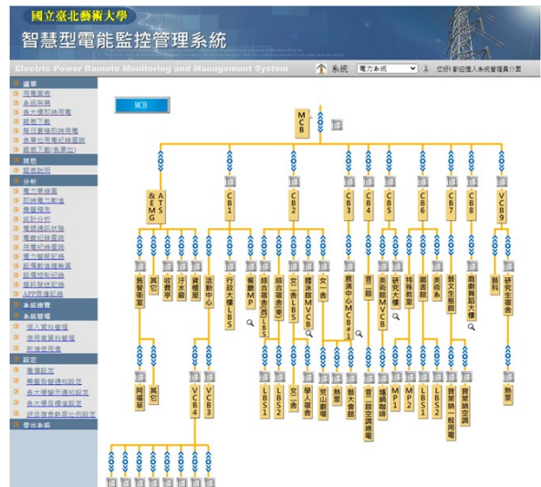
圖6 本校各大樓智慧型電能監控管理系統情形。
