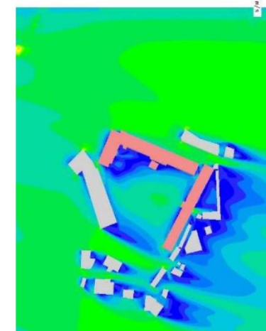
夏季氣流模擬
